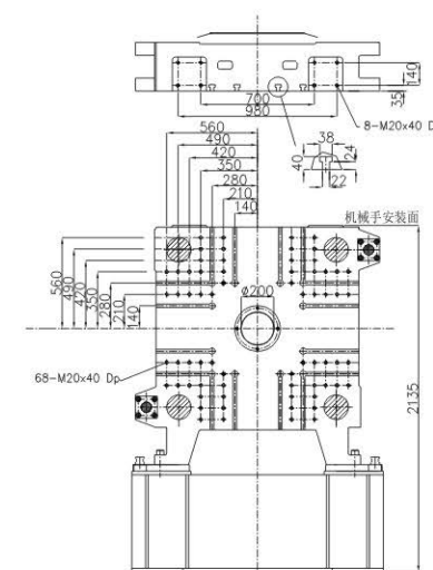
固定模板 Fixed Platen
