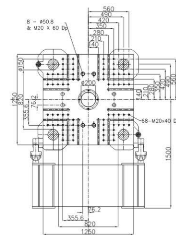
移動模板 Moving Platen
