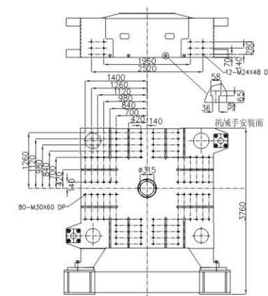
固定模板 Fixed Platen
