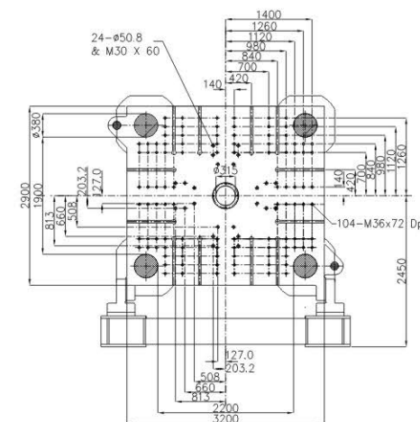
移動模板 Moving Platen
