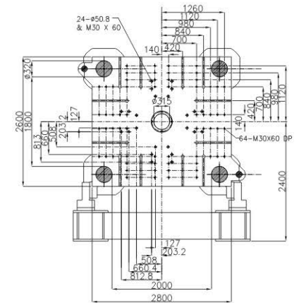
移動模板 Moving Platen
