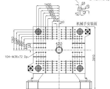
固定模板 Fixed Platen
