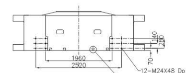
移動模板 Moving Platen
