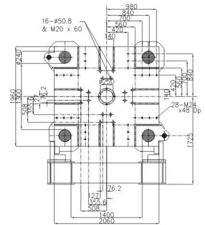
移動模板 Moving Platen
