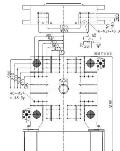
固定模板 Fixed Platen
