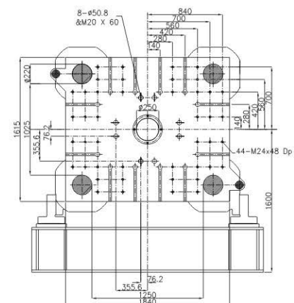
移動模板 Moving Platen
