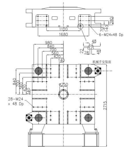
固定模板 Fixed Platen
