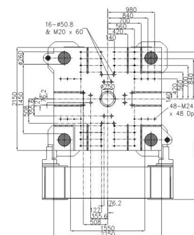
移動模板 Moving Platen
