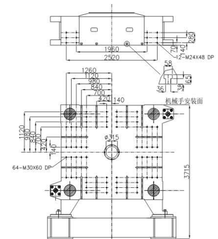
固定模板 Fixed Platen
