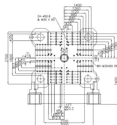
移動模板 Moving Platen
